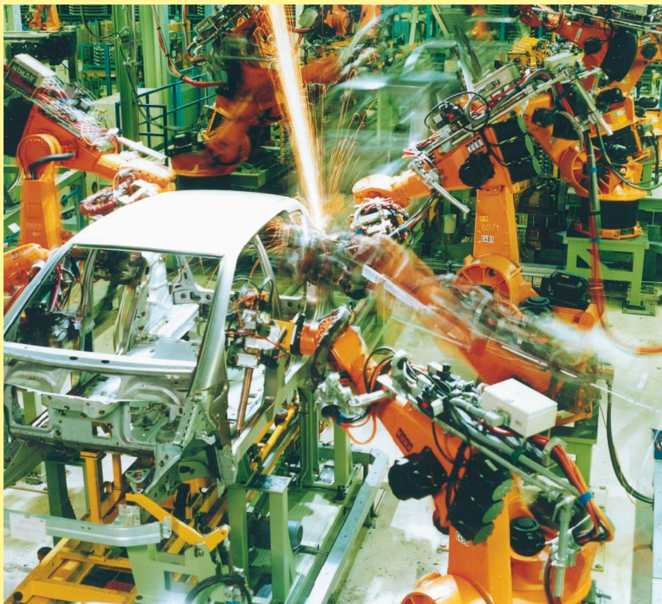
汽车生产的焊接机器人 ABB Robotics AB, Västerås, Sweden
