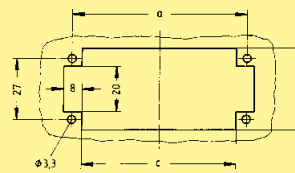
面板开孔
