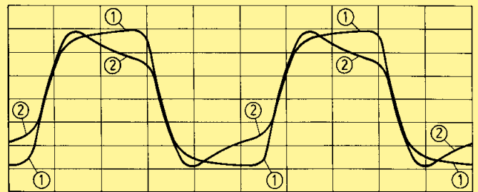
人工老化后的信号失真
