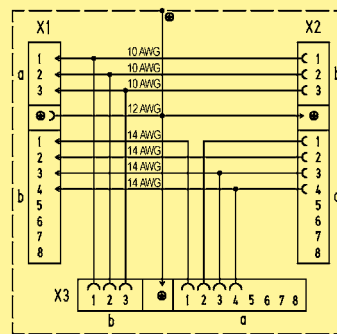
接线图
