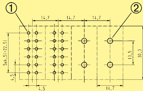
Han DD®模块
