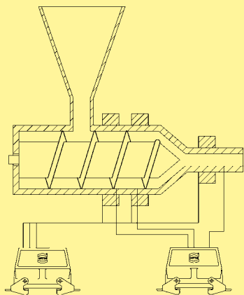
一个热回路的概况
