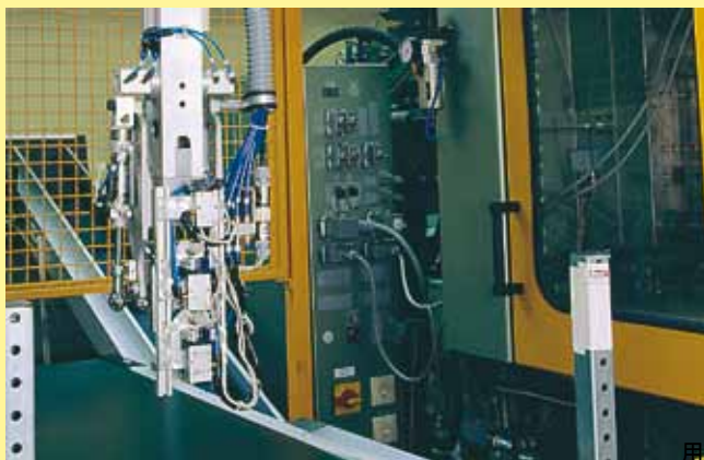
在注塑机上的连接器
