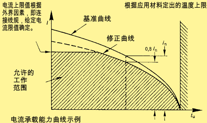
载流曲线示例
