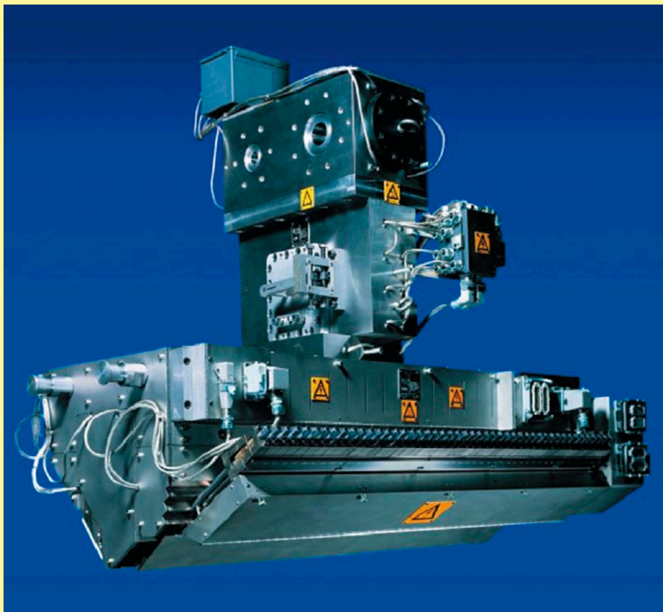
双轴取向膜模头 , Cloeren Inc., 奥兰治 (德州), 美国
